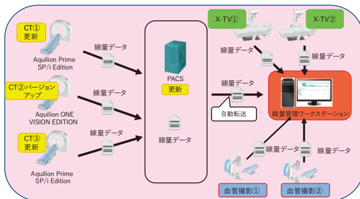
被ばく線量管理システム構成
